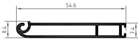
Terminal autoblocante 1000 60637
