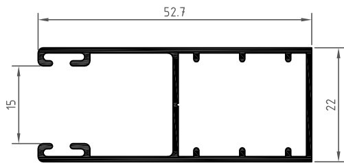
Guía H-25 50527
